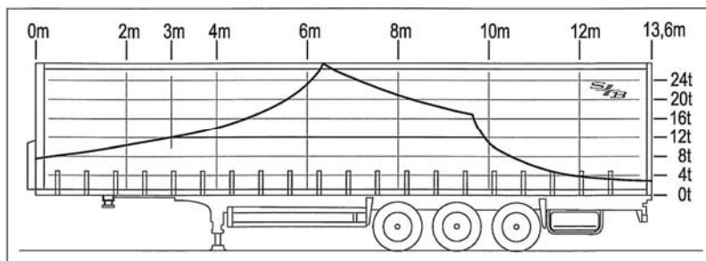
Abb. 5: Beispiel für Lastverteilungsplan eines dreiachsigen Sattelauflegers
