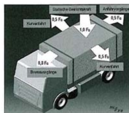
Abb. 2: Im Fahrbetrieb für die Ladungssicherung zu berücksichtigende Massenkkräfte (Quelle: VDI 2700)
