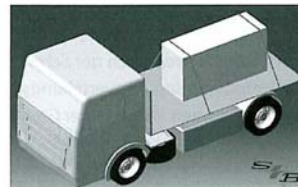
Abb. 8: Gurtverlegung beim Niederzurren (kraftschlüssige Sicherung)
