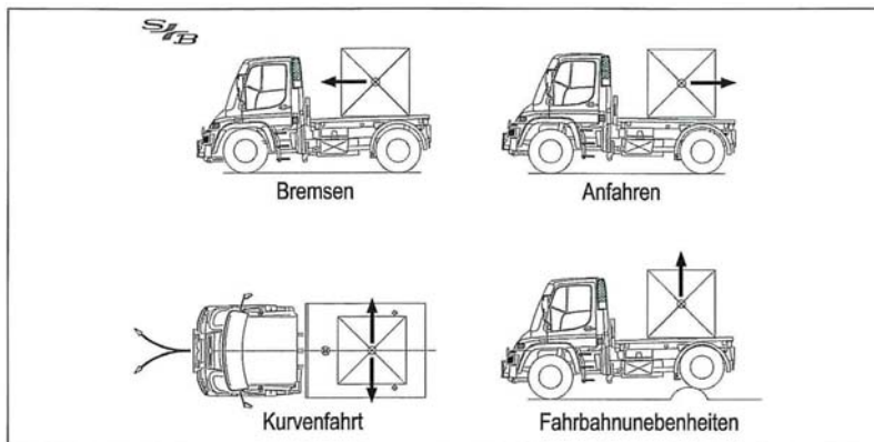
Abb. 1: Massenkräfte am Ladegut
