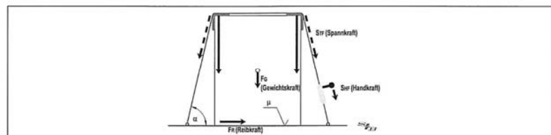
Abb. 9: Kräfte beim Niederzurren
